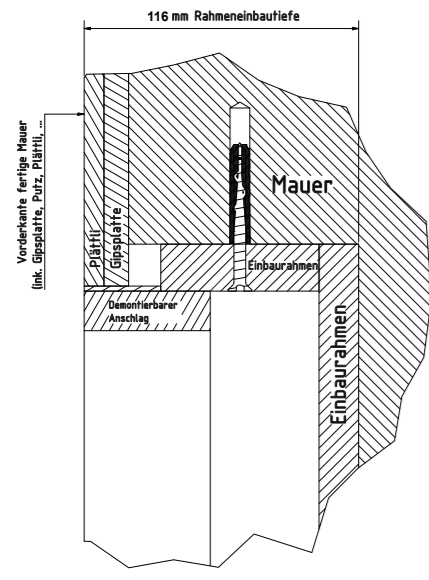
geschraubt in Vormauerung
